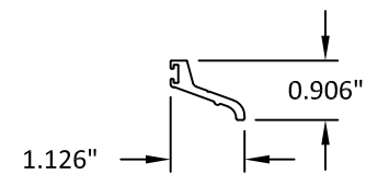
16 DOOR STOP
