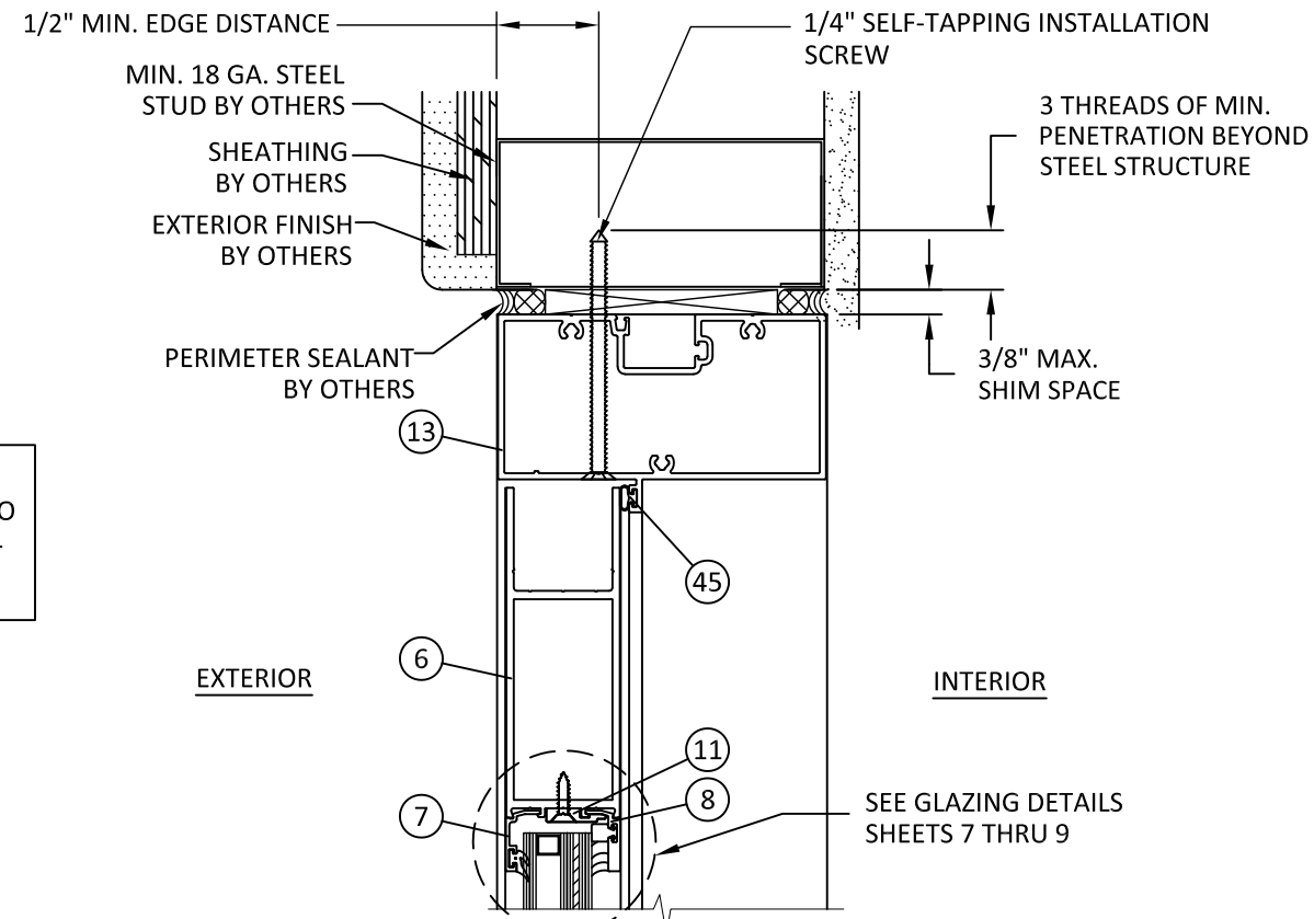
C 3 VERTICAL SECTION DOOR HEAD - STEEL STUD
